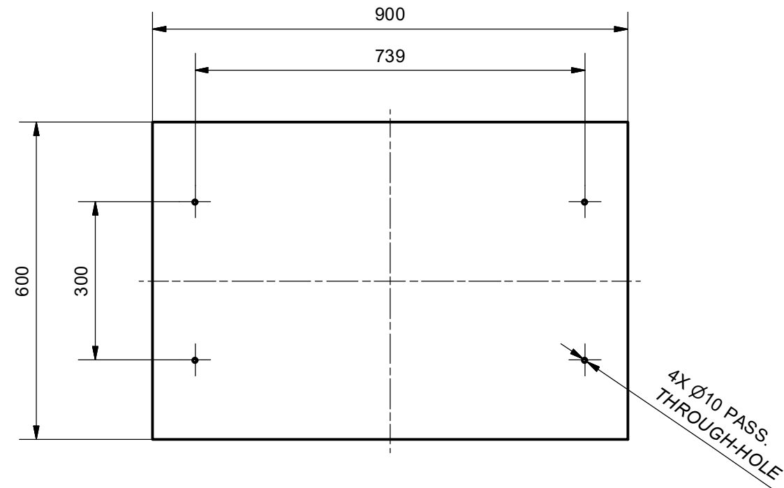
VISTA DALL'ALTO - TOP VIEW
